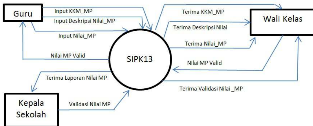
Gambar 2. Diagram konteks SIPK13
