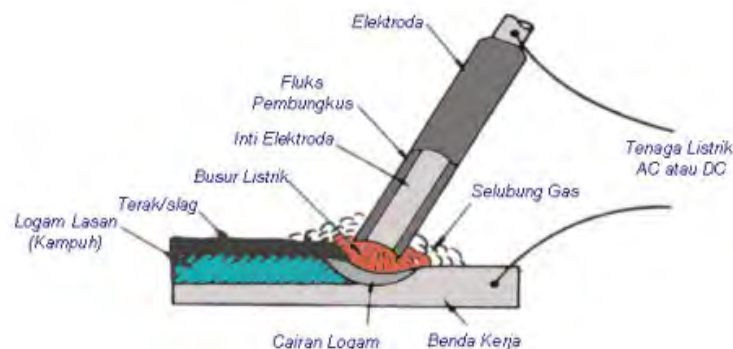
Gambar 1. Proses Pengelasan dengan elektroda terbungkus
