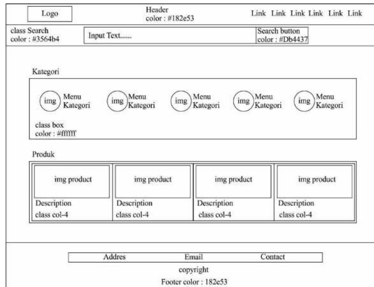
Gambar: 3.14 Interface Halaman Produk
