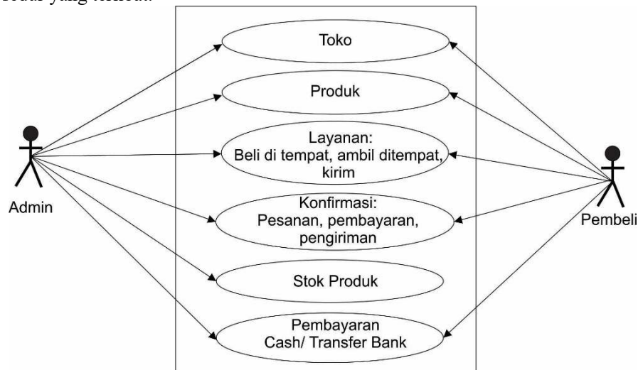
Gambar 3.1 Use Case Prosedur pembelian produk
